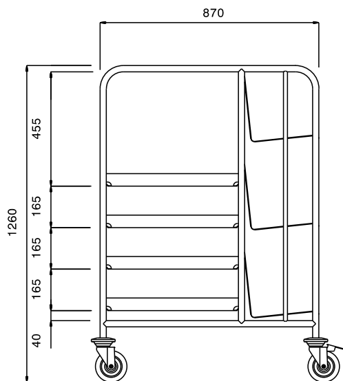
Front aanzicht
